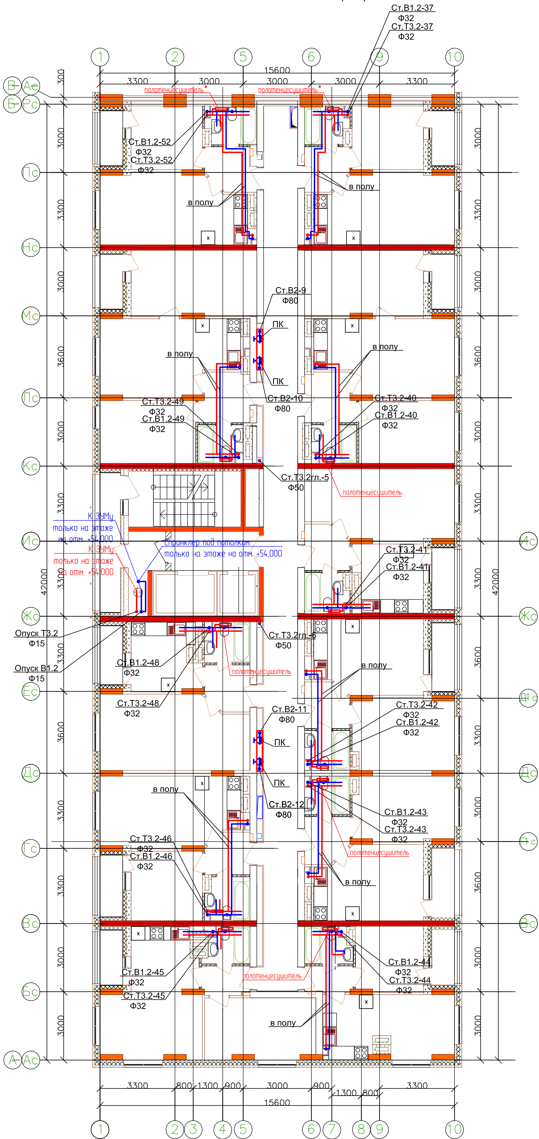
План 12-19 этажей секции в осях 1-10 и А-Б с сетями В1.2, В2, Т3.2
